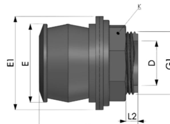
Tankadapter huiddoorvoer
